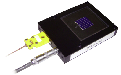
基準太陽電池セルは、I-Vテストステーションのセルホルダアセンブリにマウント可能です。
