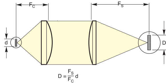
図1. ランプからの射出光を2つのレンズで平行化およびフォーカス
