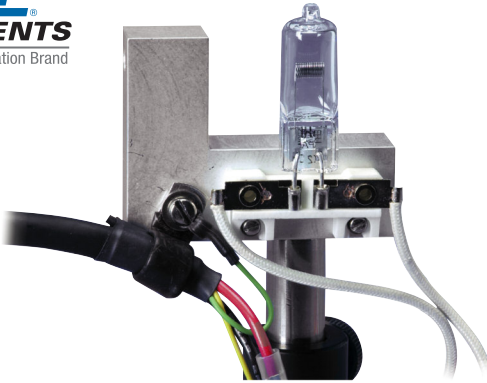
6334ランプをマウントした66306ロッドマウント
