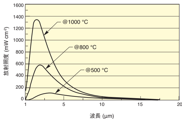
図2. Driel黒体炉の、さまざまなキャビティ温度における放射照度
